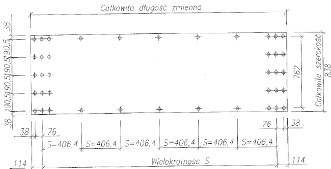
Rysunek 1 – Rzut arkusza blachy (płaszcza – wymiary przed nadaniem krzywizny). Tolerancje wymiarów: wymiarów = 406,4: (-0 mm/+3 mm)
