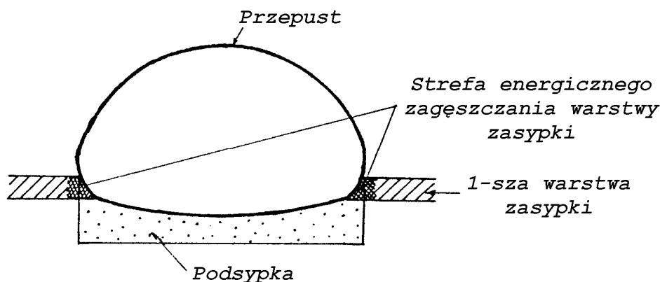
Rysunek 3 – Schemat zagęszczenia 1-szej warstwy zasyпки przepustu
