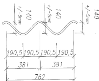
Rysunek 2 – Przekrój fali
